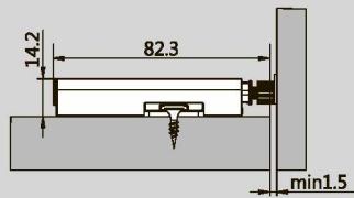
Монтаж накладного толкателя с крестообразной монтажной планкой
