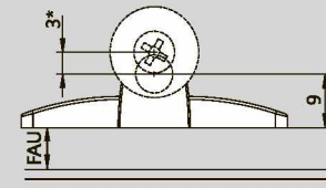
FAU-наложение фасада снизу
