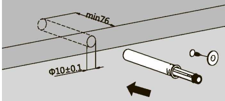
Монтаж накладного толкателя со встроенной монтажной планкой
