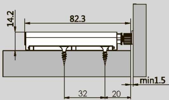
Монтаж накладного толкателя с крестообразной монтажной планкой
