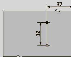
Монтаж накладного толкателя с крестообразной монтажной планкой
