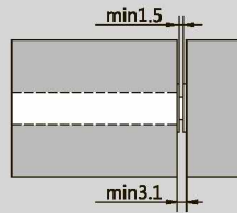
Монтаж накладного толкателя со встроенной монтажной планкой
